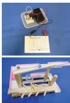
講座で作る「電子迷路装置」と「ころころスイッチ」
